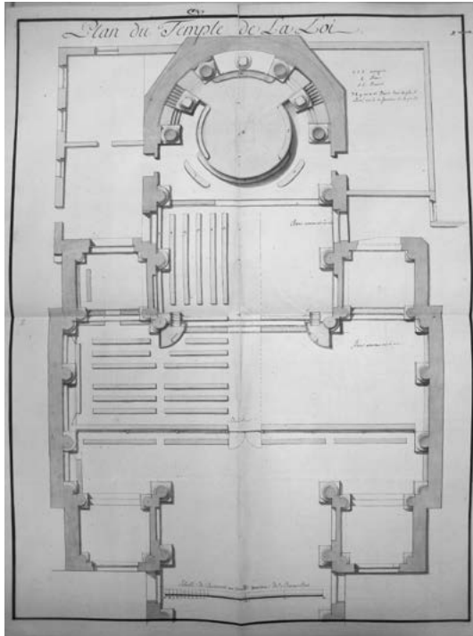
Ontwerp voor het nieuwe zaalplan van de Brusselse tempel van de Wet (1797). Tekening door Claude Fisco.
