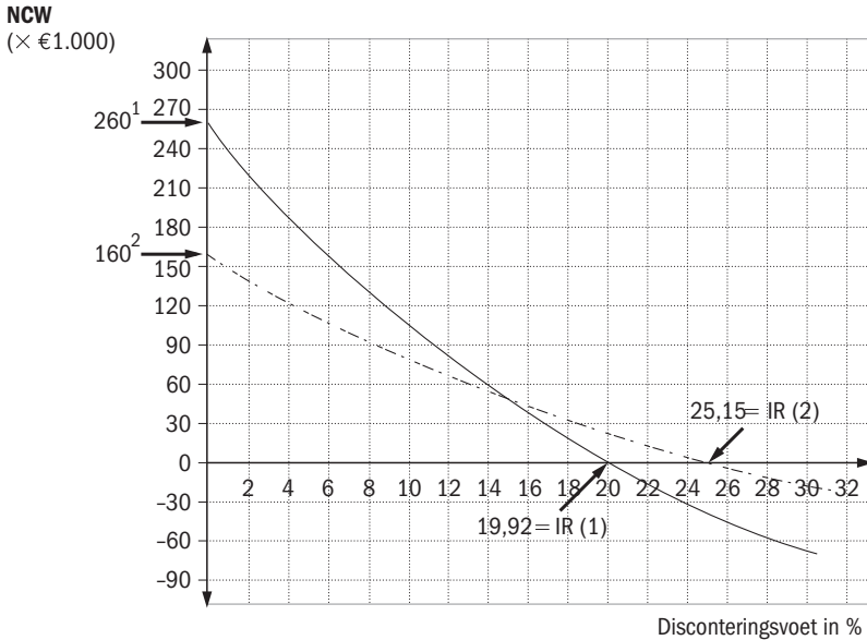
FIGUUR 1.13 Vergelijking NCW machine X en Y
