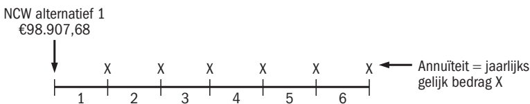
FIGUUR 1.9 Herrekening van de NCW tot een jaarlijks gelijk bedrag X (alternatief 1)
